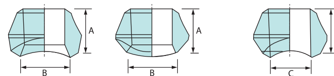
Weldolet redukovaný ASME B16.25
